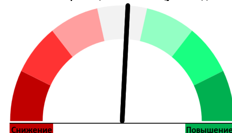
Снижение/рост цен на пшеницу на 14 дней
